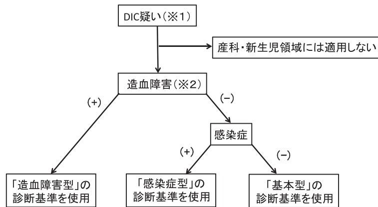
図1 DIC診断基準適用のアルゴリズム
